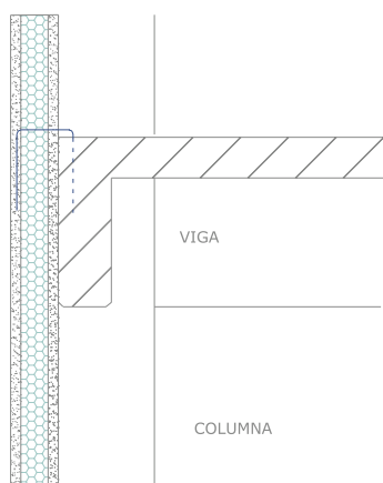
ALTERNATIVA: GANCHOS OCULTOS EN CONTRAPISO. (EVITA OCULTAMIENTO DE GANCHO EN CIELORRASO)
