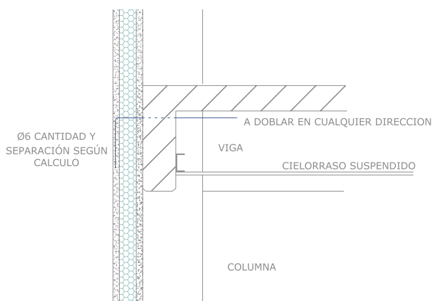
ALTERNATIVA: GANCHOS OCULTOS EN CIELORRASO SUSPENDIDO
